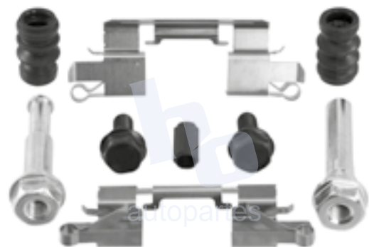
KIT DE CALIPER RUEDA DELANTERA CHEVROLET CITY EXPRESS (15-18) 8200 D1094, NISSAN FRONTIER (05-15) 8200 D1094, 8200 D1900, LEAF (10-17) 8200 D1900, 8757 D1548, NAVARA (03-09) 8200 D1094, NP300 (15) 8200 D1900, NV200 (13-17) 8200 D1094, PATHFINDER (05-14), XTERRA (05-16) 8200 D1094, 8200 D1900.
