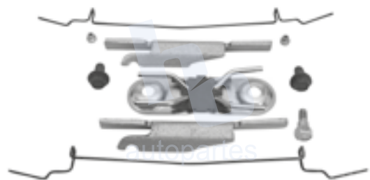
KIT DE CALIPER RUEDA DELANTERA FORD F700 (83-97), F800 (83-97), F900 LN 700-800 (83-97), F900 LT 800-900 (83-97) 7809 D236.
