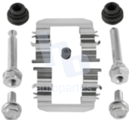
KIT DE CALIPER RUEDA DELANTERA KIA SOUL (14-16) 8505 D1397.
