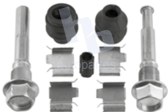
KIT DE CALIPER RUEDA DELANTERA KIA SPORTAGE (93-06) 7641 D774.
