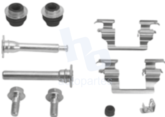
KIT DE CALIPER RUEDA DELANTERA TOYOTA COROLLA (98-02) 7611 D741.
