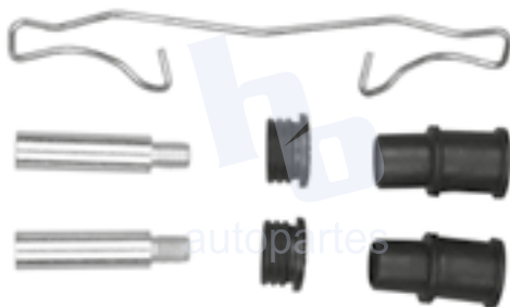
KIT DE CALIPER RUEDA DELANTERA RENAULT CAPTURE 2.0L (16-19), DUSTER (12-16), FLUENCE (11-13), OROCH (16-19) 8844 D1627.
