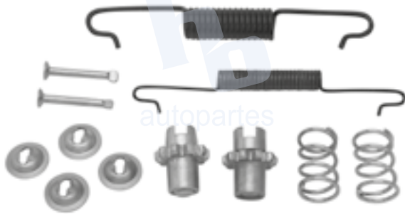
KIT PARA FRENO DE TAMBOR RUEDA DELANTERA VOLKSWAGEN 1500 (73-94), 1600 (73-94) 881A 269.
