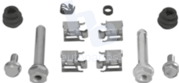
KIT DE CALIPER RUEDA DELANTERA TOYOTA COROLLA (00-19) 8845 D1628, 8331 D1211, MATRIX (09-13), RAV4 (06-18) 8331 D1211, PRIUS C (11-16), YARIS (05-16) 8845 D1628.
