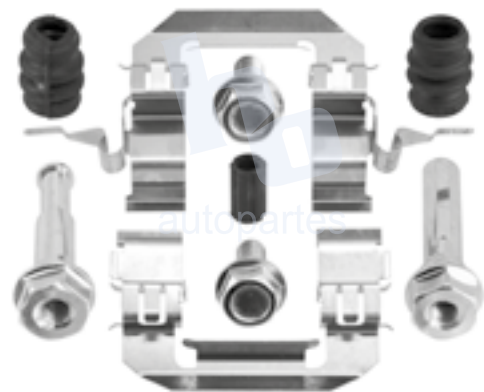
KIT DE CALIPER RUEDA DELANTERA MAZDA CX5 (13-17) 8836 D1623, NISSAN JUKE (14-17), MAXIMA (09-18), ROGUE (08-17), SENTRA (07-12) 8836 D1374.
