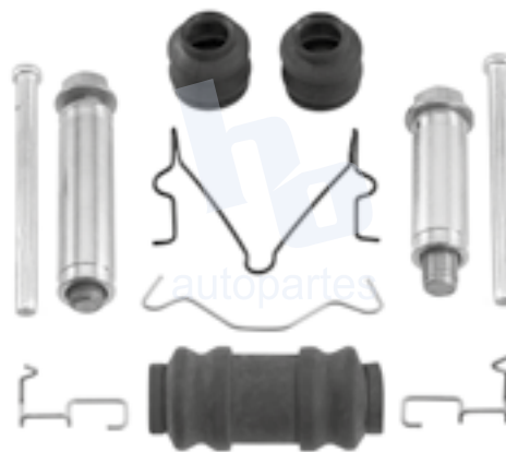
KIT DE CALIPER RUEDA TRASERA MITSUBISHI MONTERO 4WD (97-04) 7602 D733.
