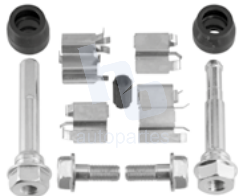
KIT DE CALIPER RUEDA DELANTERA TOYOTA RAV4 (01-05) 7738 D862.
