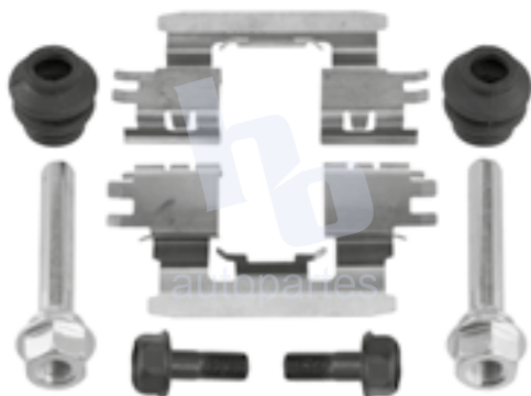
KIT DE CALIPER RUEDA DELANTERA SUZUKI AERIO (02-07) 7839 D937.
