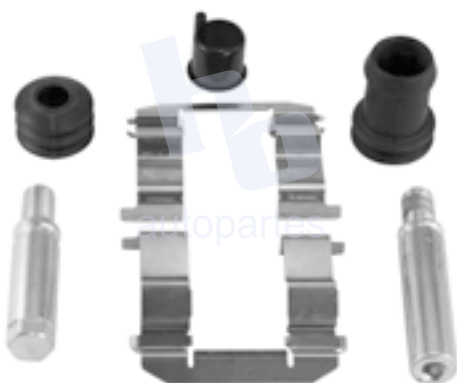
KIT DE CALIPER RUEDA DELANTERA MAZDA PROTEGE (99-00) 7515 D637.
